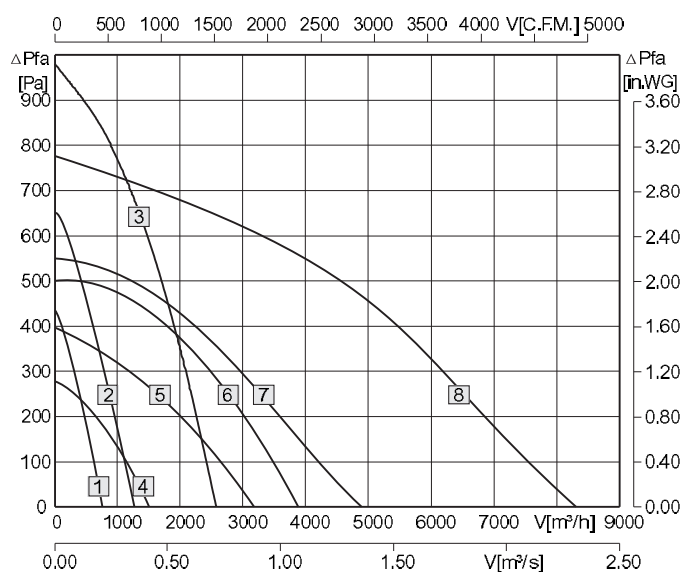
KHA_管道风机快速选型图表:
