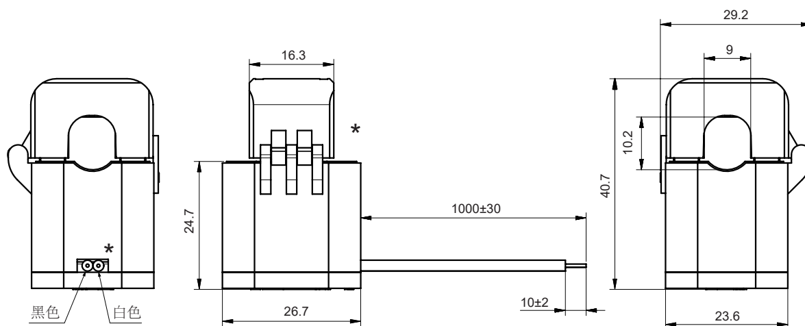
外形图
